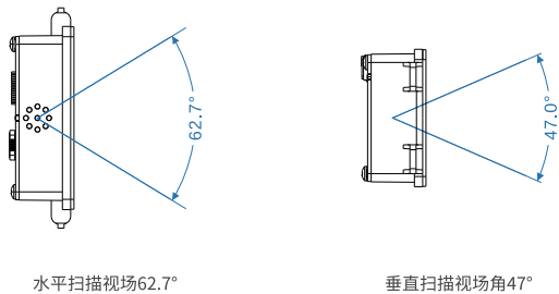
XL-3042mini扫描视场角度图
