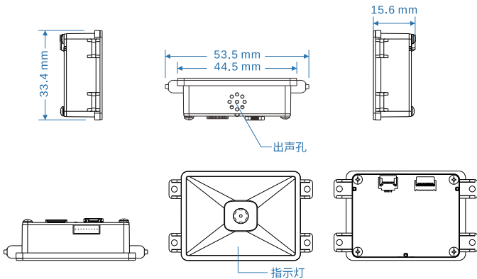
XL-3042mini尺寸图
