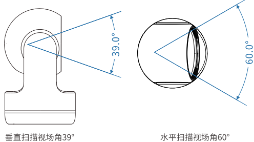
XL-2610A扫描视场角度图
