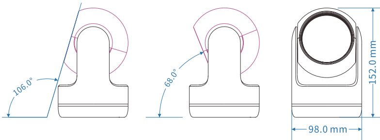
XL-2610A尺寸图
