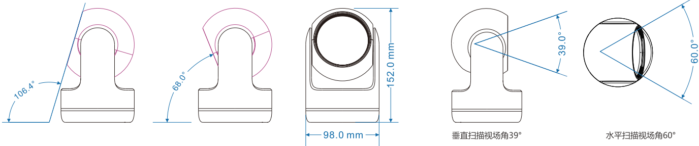
XL-2610尺寸图
